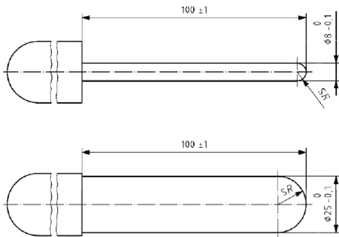
Рисунок 7 — Конусообразный щуп
